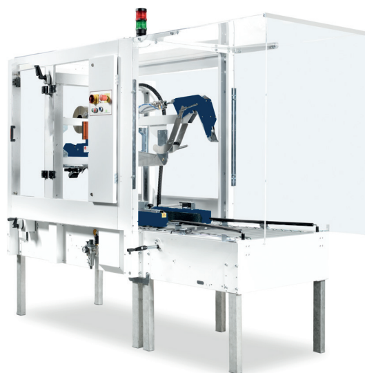
CT 303 SDF med centreringsenhet (tillval)
